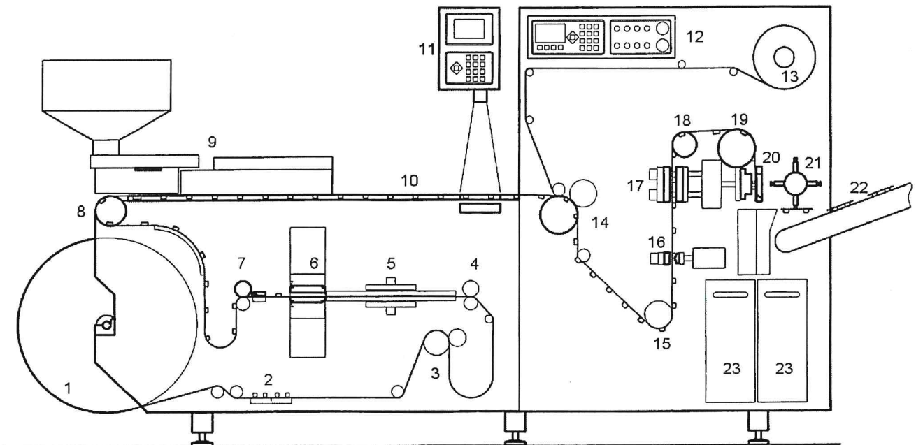
Bild 2.6.1 Maschinenübersicht
